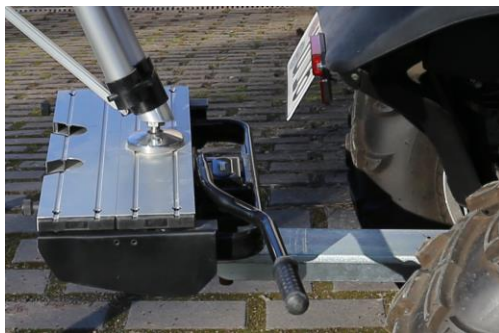
Die Verlängerung der Anhängerkupplung und die daran angekoppelte Stativhalterung.
